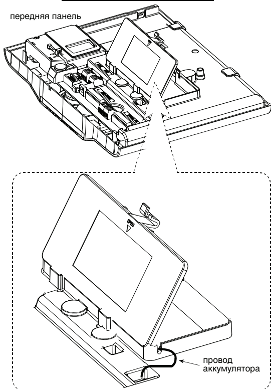
Рисунок 10. Замена аккумулятора
